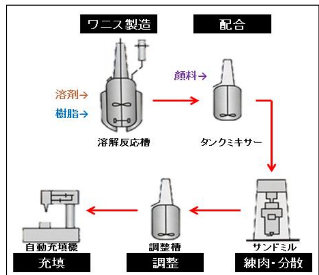
図2 製造工程の製造プロセス
